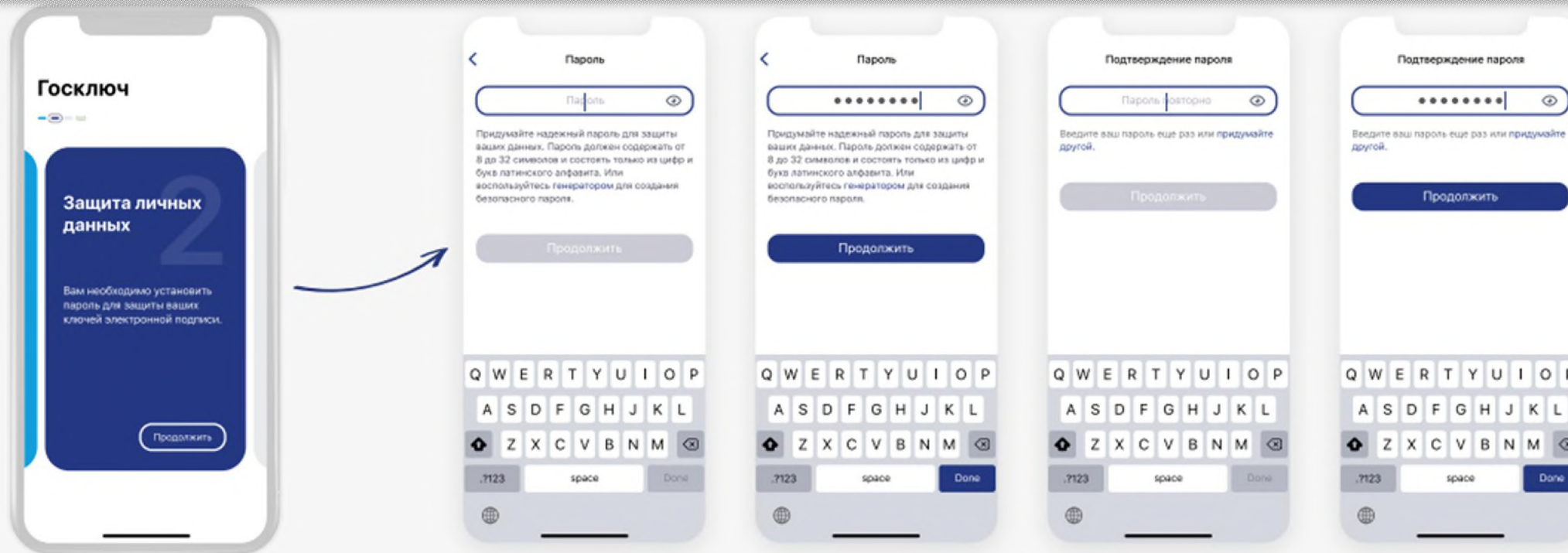
1.6 Устанавливаем пароль
